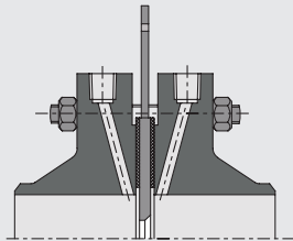
Угловой патрубок для отбора давления
