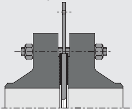
Выступающая поверхность
