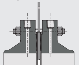
Фланцевый патрубок для отбора давления
