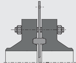
Уплотнительное кольцо
