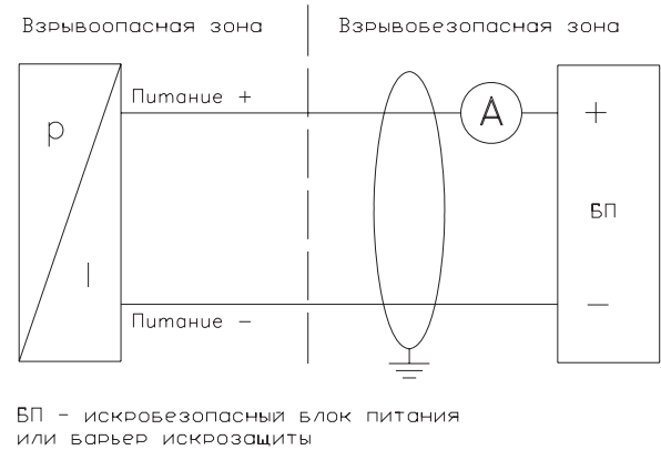
Рисунок В.2 – Схема внешних электрических соединений датчиков взрывозащищенного исполнения.
