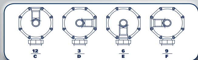
P143, положение сбросного отверстия
