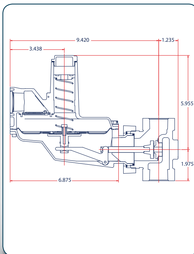
Габаритные размеры, P143 (дюймы)
